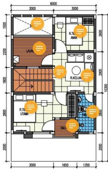
DENAH LT. SKALA 1 : 100
