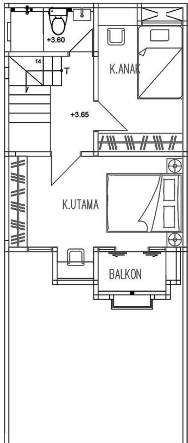
LANTAI 2
