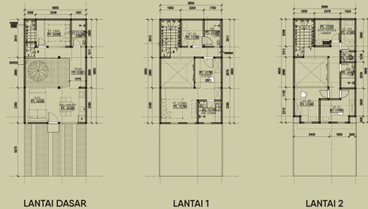
LANTAI DASAR
