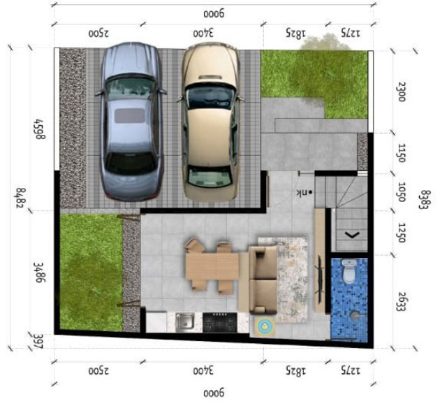
DENAH LANTAI 1 LEBAR 9 METER SKALA: 1:100
