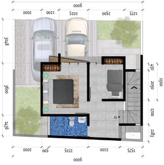
DENAH LANTAI 2 LEBAR 9 METER SKALA: 1:100
